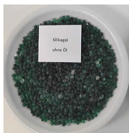
Abbildung 4: Silicagel vor und nach der Regeneration. Links ohne Öl, rechts mit Öl.
