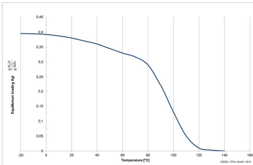
Abbildung 1: Gleichgewichtsbeladung von Silicagel in Abhängigkeit der Temperatur.
